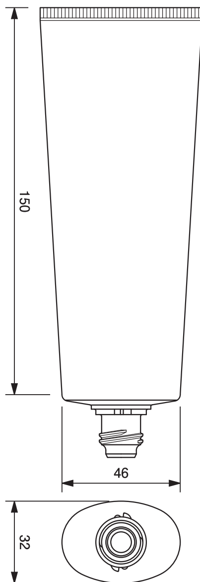
40φオーバルチューブ -147.8 40mm dia. Oval Tube-147.8
