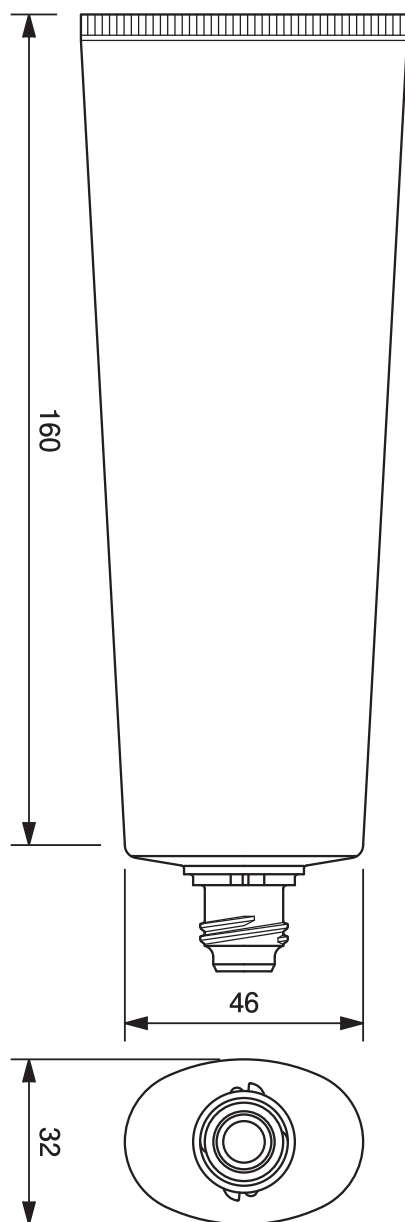
40φオーバルチューブ -160.3 40mm dia. Oval Tube-160.3
