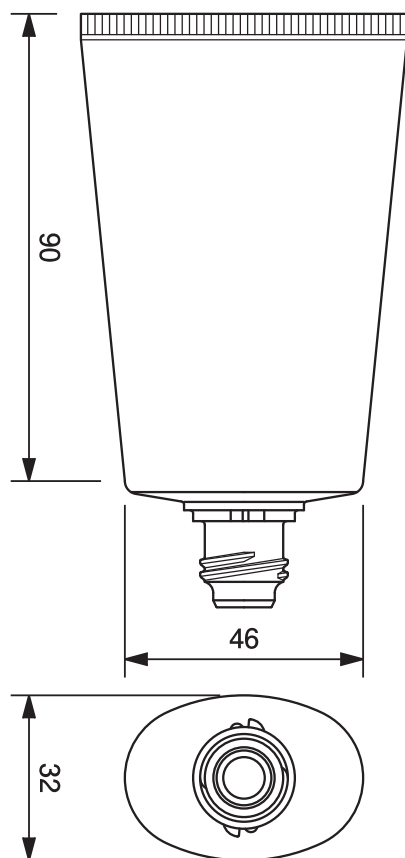
40φオーバルチューブ -75 40mm dia. Oval Tube-75
