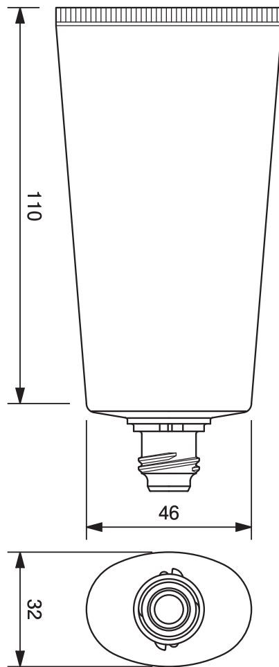
40φオーバルチューブ -98.6 40mm dia. Oval Tube-98.6
