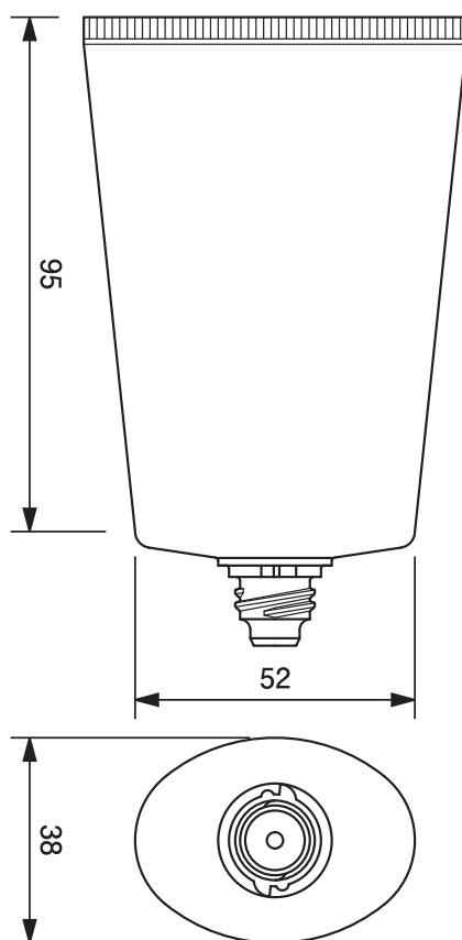
45φオーバルチューブ -102.7 45mm dia. Oval Tube-102.7
