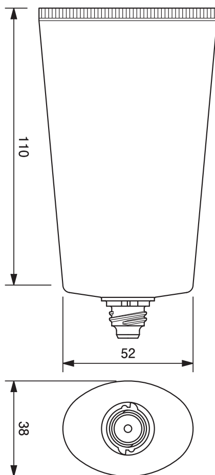
45φオーバルチューブ -124.2 45mm dia. Oval Tube-124.2
