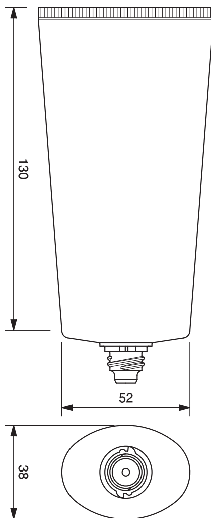
45φオーバルチューブ -153.9 45mm dia. Oval Tube-153.9
