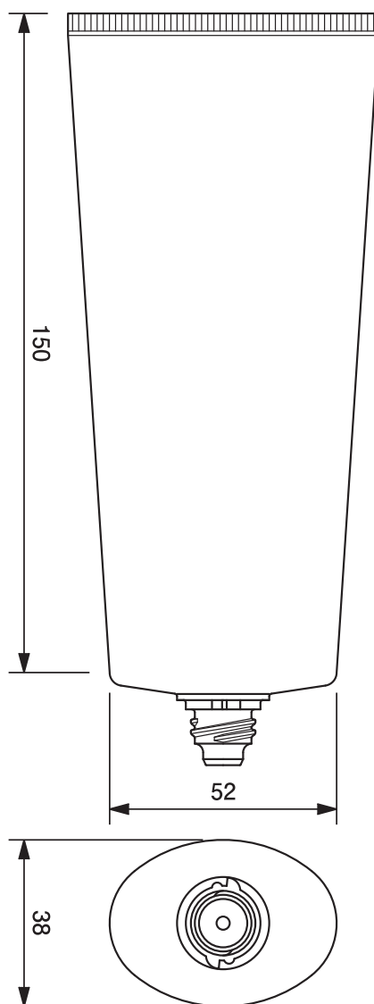
45φオーバルチューブ -186.3 45mm dia. Oval Tube-186.3
