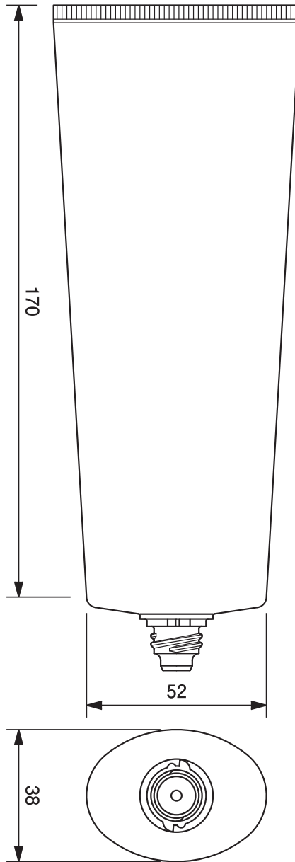
45φオーバルチューブ -217 45mm dia. Oval Tube-217
