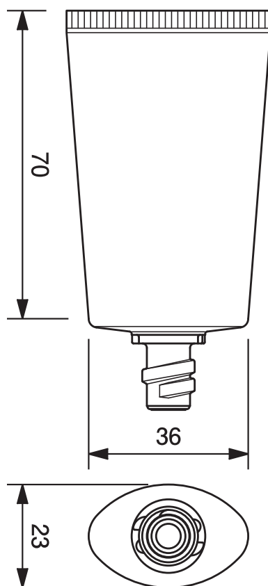
30φオーバルワンタッチチューブ -30.7 30mm dia. Oval Flip-top Cap Tube-30.7
