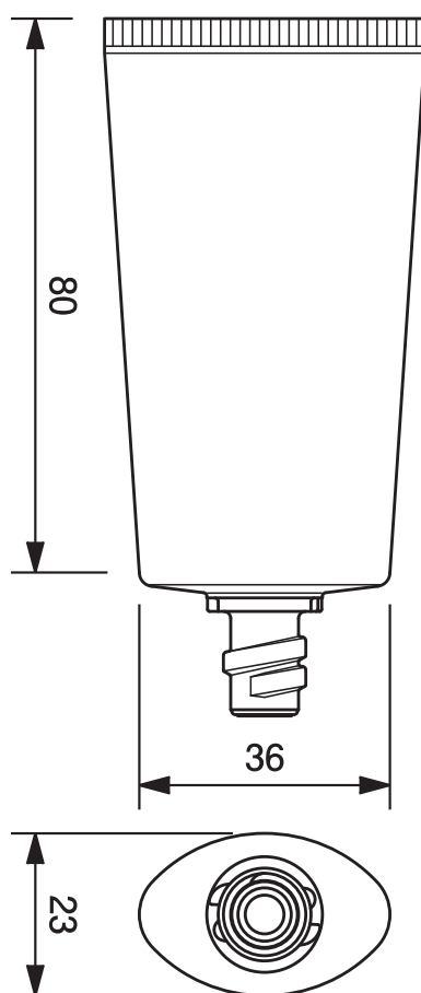
30φオーバルワンタッチチューブ -35.8 30mm dia. Oval Flip-top Cap Tube-35.8
