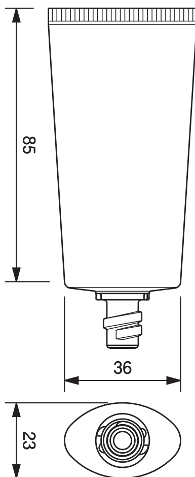
30φオーバルワンタッチチューブ -39.7 30mm dia. Oval Flip-top Cap Tube-39.7
