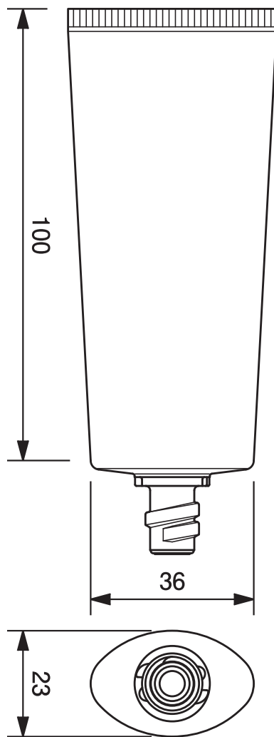
30φオーバルワンタッチチューブ -49.5 30mm dia. Oval Flip-top Cap Tube-49.5
