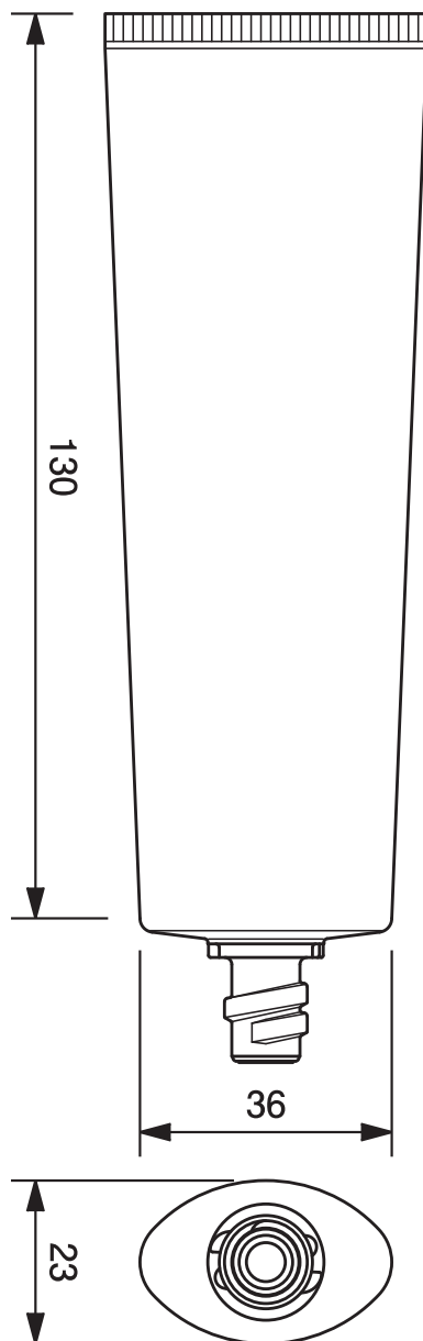
30φオーバルワンタッチチューブ -70.7 30mm dia. Oval Flip-top Cap Tube-70.7
