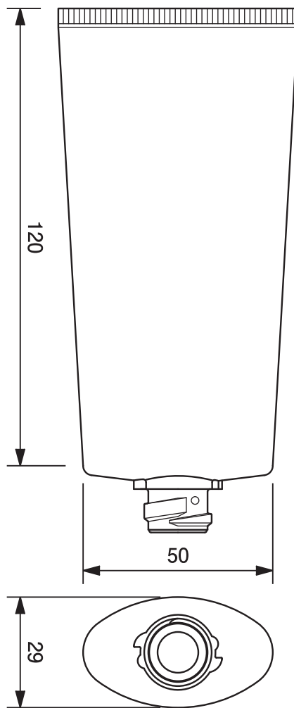
40φオーバルワンタッチチューブ -109.4 40mm dia. Oval Flip-top Cap Tube-109.4
