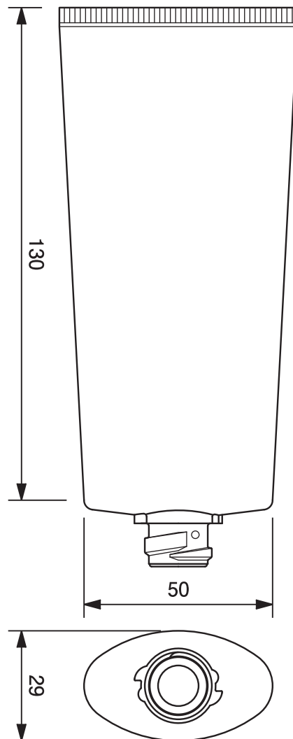
40φオーバルワンタッチチューブ -122.2 40mm dia. Oval Flip-top Cap Tube-122.2
