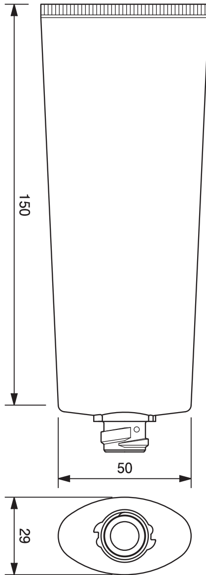
40φオーバルワンタッチチューブ -147.8 40mm dia. Oval Flip-top Cap Tube-147.8
