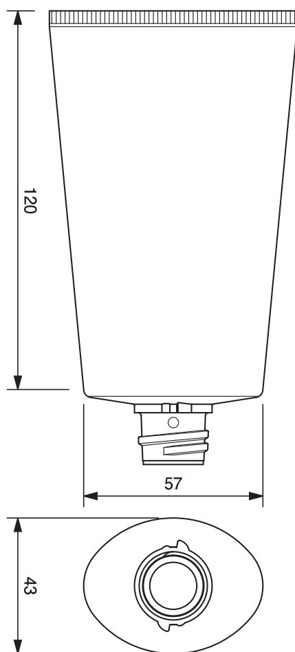
50φオーバルワンタッチチューブ -164.1 50mm dia. Oval Flip-top Cap Tube-164.1
