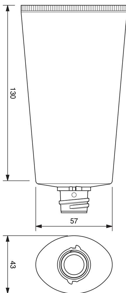
50φオーバルワンタッチチューブ -176.8 50mm dia. Oval Flip-top Cap Tube-176.8
