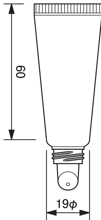
19φグロスチューブ -11.9 19mm dia. Gloss Tube-11.9
