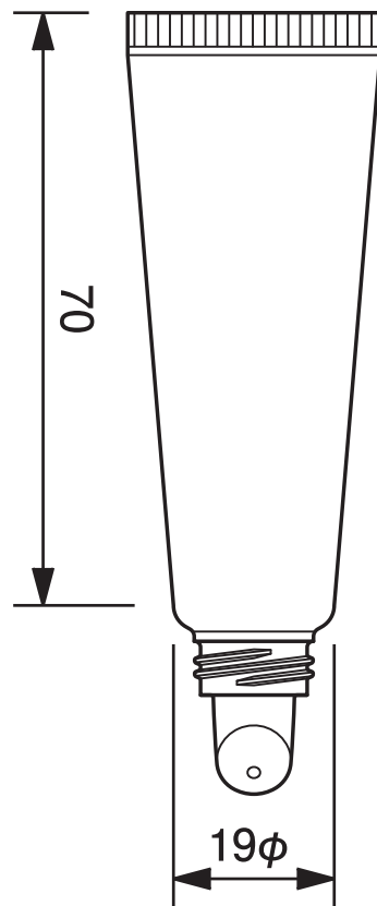
19φグロスチューブ -14.3 19mm dia. Gloss Tube-14.3
