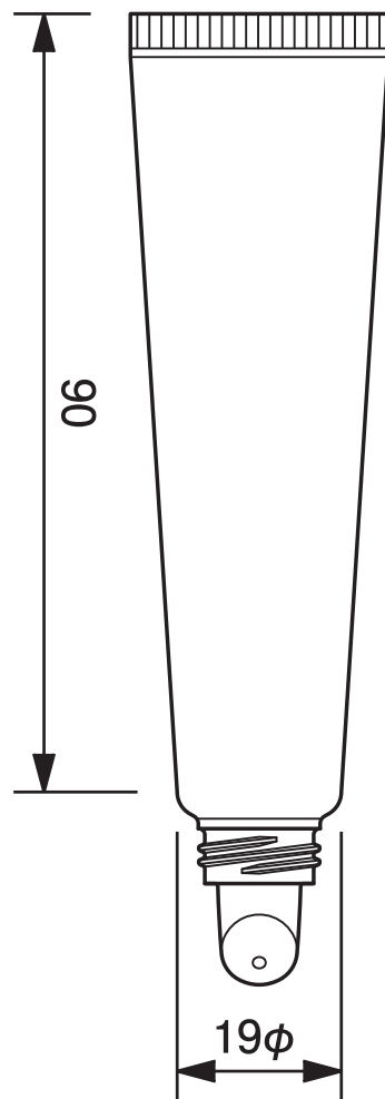
19φグロスチューブ -19.6 19mm dia. Gloss Tube-19.6
