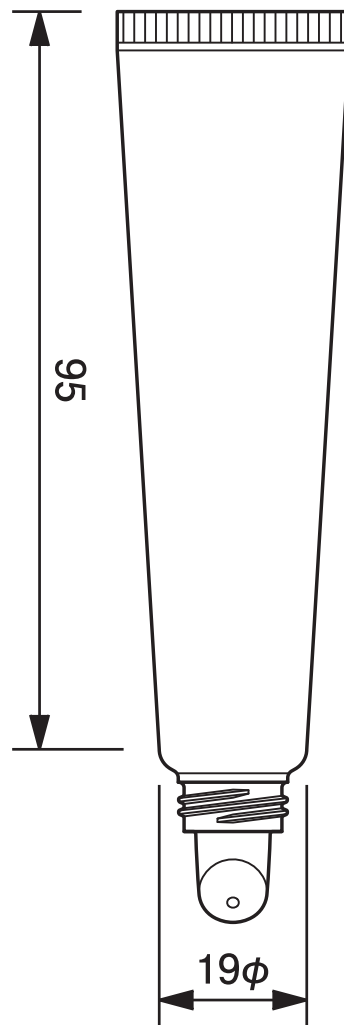
19φグロスチューブ -20.7 19mm dia. Gloss Tube-20.7
