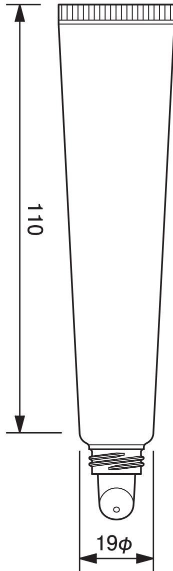
19φグロスチューブ -24.5 19mm dia. Gloss Tube-24.5
