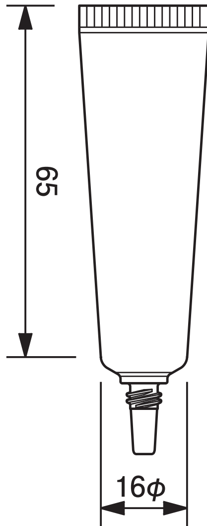
16φノズルチューブ -10 16mm dia. Nozzle Tube-10
