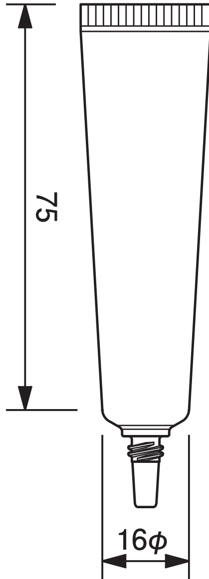
16φノズルチューブ -12 16mm dia. Nozzle Tube-12
