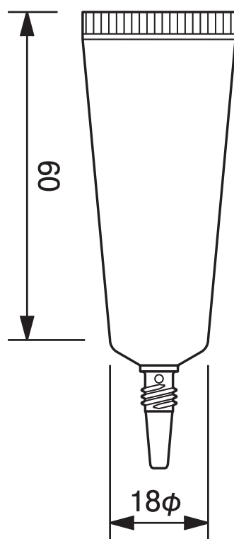
18φノズルチューブ -10.5 18mm dia. Nozzle Tube-10.5
