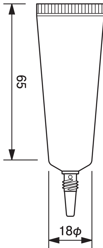
18φノズルチューブ -11.6 18mm dia. Nozzle Tube-11.6
