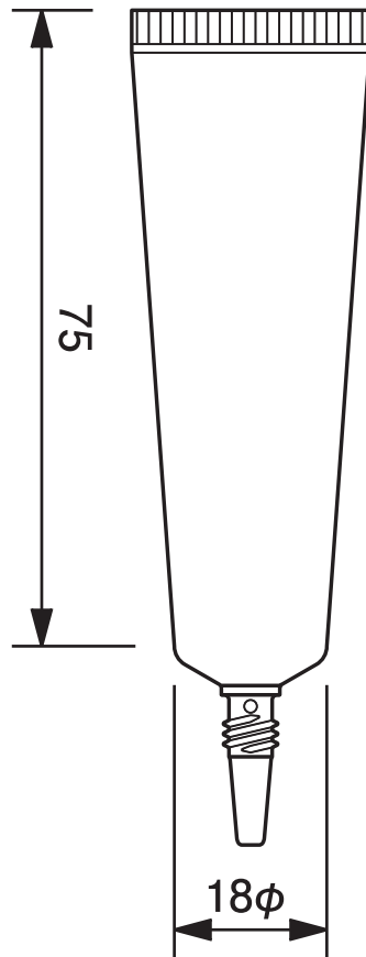
18φノズルチューブ -14.2 18mm dia. Nozzle Tube-14.2
