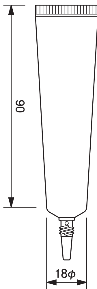
18φノズルチューブ -17.4 18mm dia. Nozzle Tube-17.4
