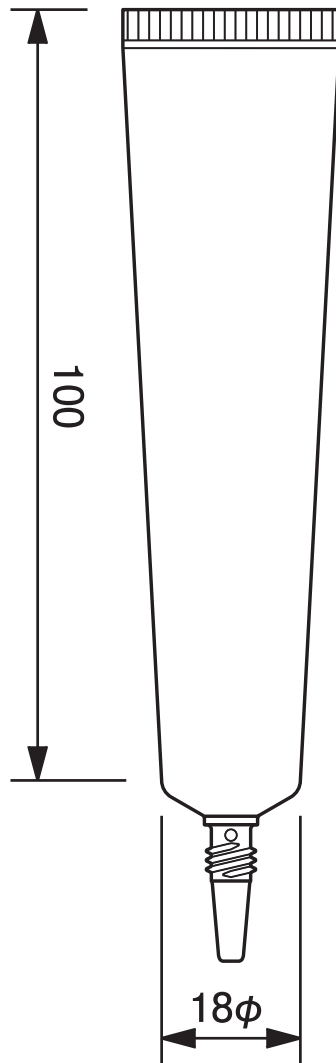
18φノズルチューブ -19.8 18mm dia. Nozzle Tube-19.8
