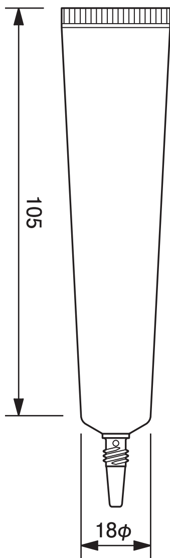
18φノズルチューブ -21 18mm dia. Nozzle Tube-21
