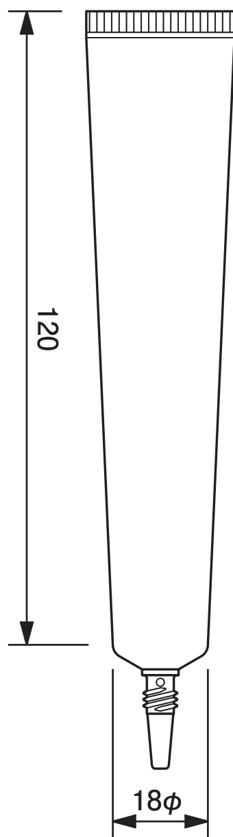
18φノズルチューブ -24.4 18mm dia. Nozzle Tube-24.4
