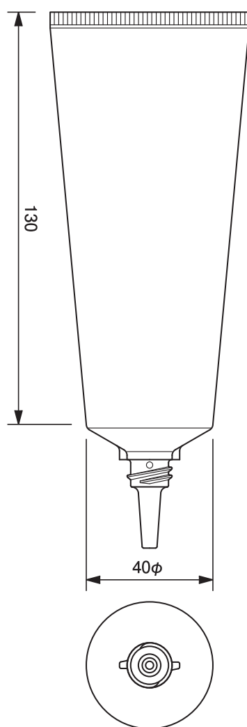
40φトンガリノズルチューブ -108.6 40mm dia. Nozzle Tube-108.6
