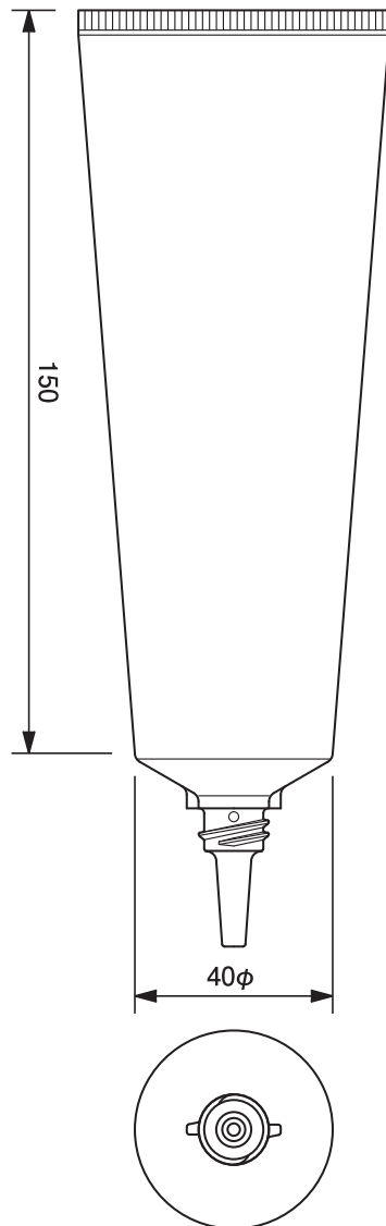
40φトンガリノズルチューブ -132.2 40mm dia. Nozzle Tube-132.2
