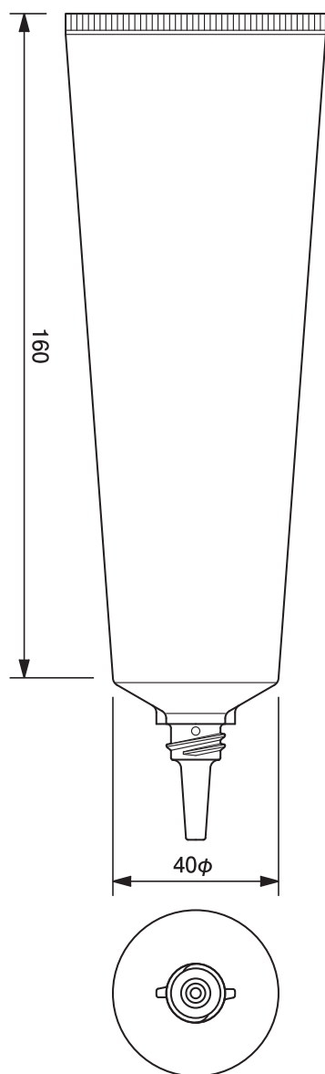
40φトンガリノズルチューブ -144 40mm dia. Nozzle Tube-144
