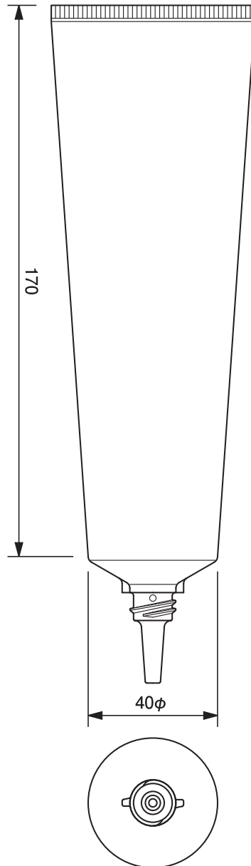
40φトンガリノズルチューブ -155.8 40mm dia. Nozzle Tube-155.8
