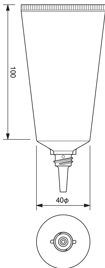
40φトンガリノズルチューブ -73.2 40mm dia. Nozzle Tube-73.2
