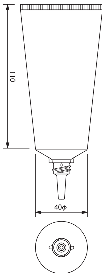
40φトンガリノズルチューブ -85 40mm dia. Nozzle Tube-85
