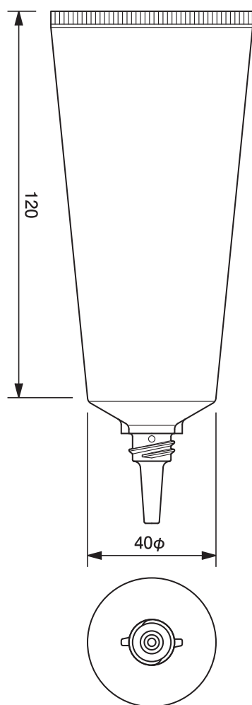
40φトンガリノズルチューブ -96.8 40mm dia. Nozzle Tube-96.8
