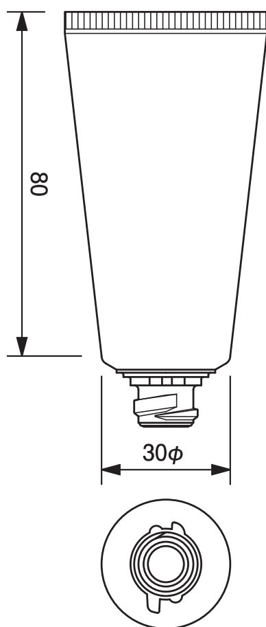
30φワンタッチチューブ -38.4 30mm dia. Flip-top Cap Tube-38.4
