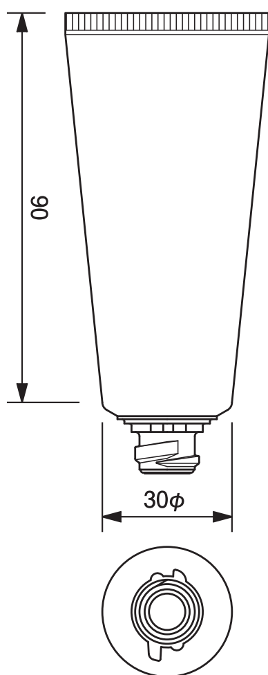
30φワンタッチチューブ -44.8 30mm dia. Flip-top Cap Tube-44.8
