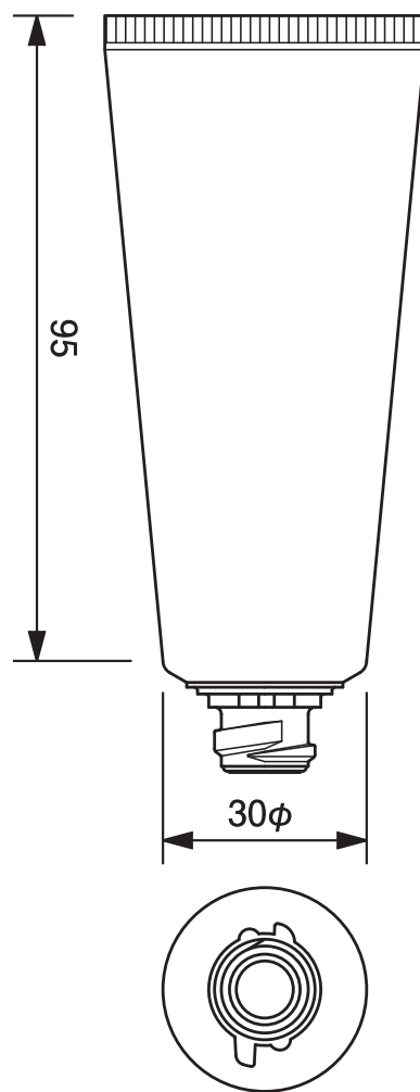
30φワンタッチチューブ -48.1 30mm dia. Flip-top Cap Tube-48.1
