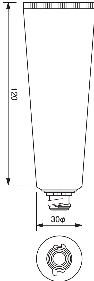
30φワンタッチチューブ -66.3 30mm dia. Flip-top Cap Tube-66.3
