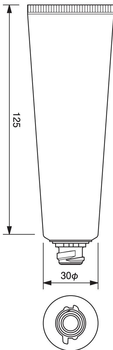
30φワンタッチチューブ -67.8 30mm dia. Flip-top Cap Tube-67.8
