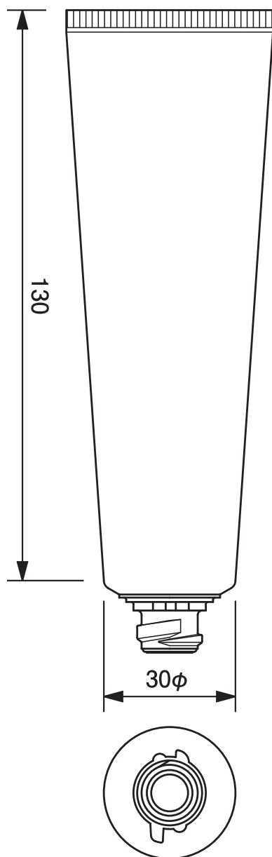
30φワンタッチチューブ -71.8 30mm dia. Flip-top Cap Tube-71.8
