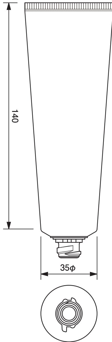
35φワンタッチチューブ -107.6 35mm dia. Flip-top Cap Tube-107.6
