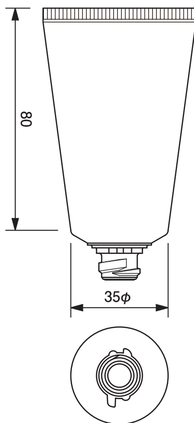
35φワンタッチチューブ -52.3 35mm dia. Flip-top Cap Tube-52.3
