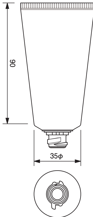
35φワンタッチチューブ -61.5 35mm dia. Flip-top Cap Tube-61.5
