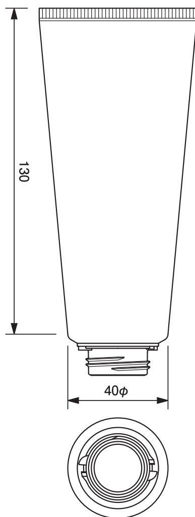
40φワンタッチチューブ -124.6 40mm dia. Flip-top Cap Tube-124.6
